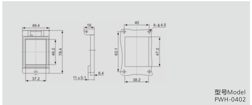
窗口产品外形尺寸、安装孔及孔位图
